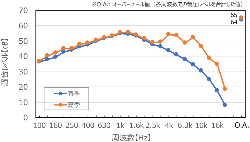
図 測定時期による周波数特性（諏訪梅林増圧ポンプ場、昼間）
